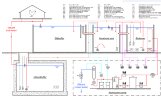
Schema 2: Schematisch overzicht van de opbouw van het waterzuiveringssysteem.
